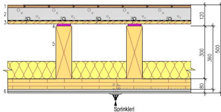
Kuva 13. Välipohjatyyppi VP801KRL (RunkoPES 2.0.). Kirjoittajan huomio: Rakennerratkaisu sisältää sprinklerin. Suomen rakentamismääräyskokoelman E1 "Rakennusten paloturvallisuus" mukaisesti automaattinen sammutusjärjestelmä on pakollinen yli kaksikerroksisissa puurakennuksissa. (Finnish Wood Research, 2013.)
