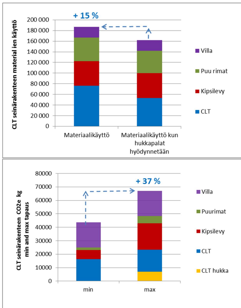
Kuva 17. Materiaalien käyttö ja kasviuonekaasupäästöt tilaelementtien seinärakenteiden valmistuksessa, tapauksessa jossa jätemateriaalit hyödynnetään tai ei. Kuvassa b lisäksi materiaalien valmistus on ollut perustapausta (min) ympäristöä kuormittavampi (max).
