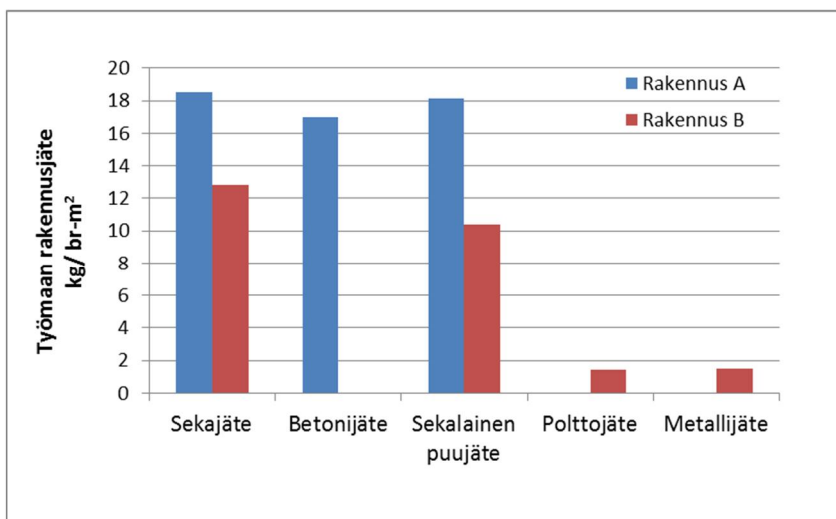
Kuva 18. Työmaajätteiden suhteelliset osuudet sekä kokonaismäärät tapaustutkimuksissa.
