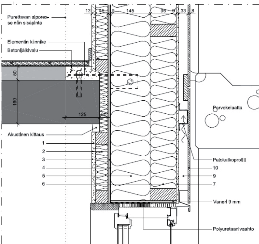
DET 6
